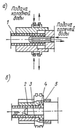
Рис. 17. Схема формования утолщенную бурта на конце трубы
