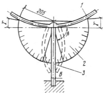
Рис. 20. Схема испытания пластмассовых труб на статический изгиб
