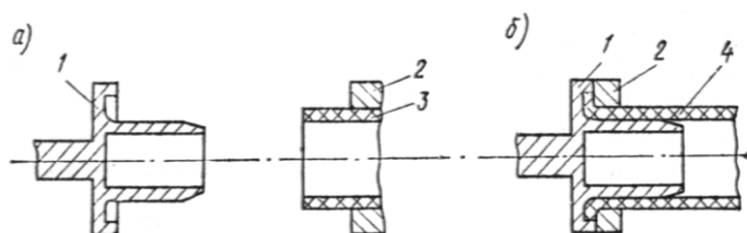
Рис. 16. Схема формирования отбортовки
