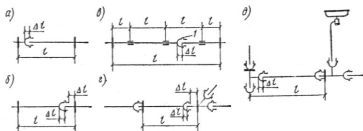
Рис. 15. Варианты расстановки креплений на канализационном трубопроводе
